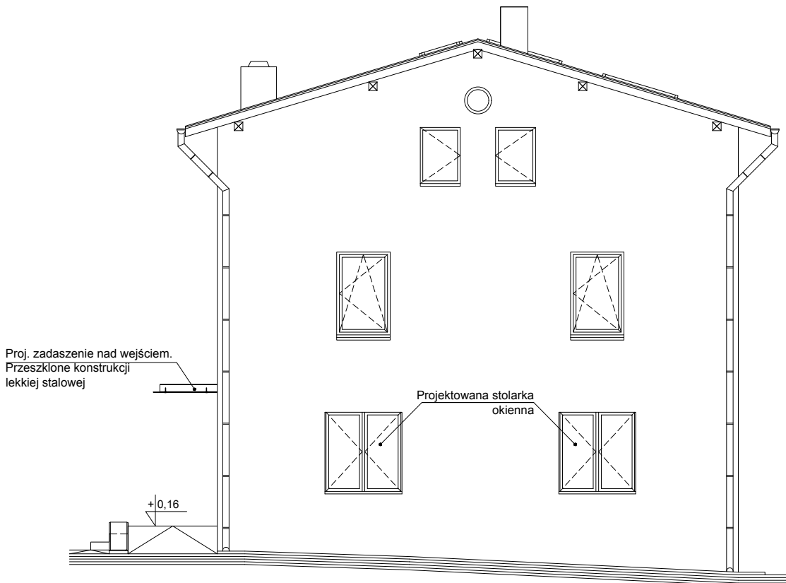
ELEWACJA POŁUDNIOWO-ZACHODNIA
