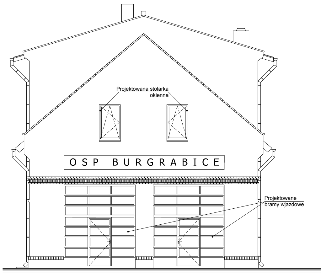
ELEWACJA PÓŁNOCNO-WSCHODNIA
