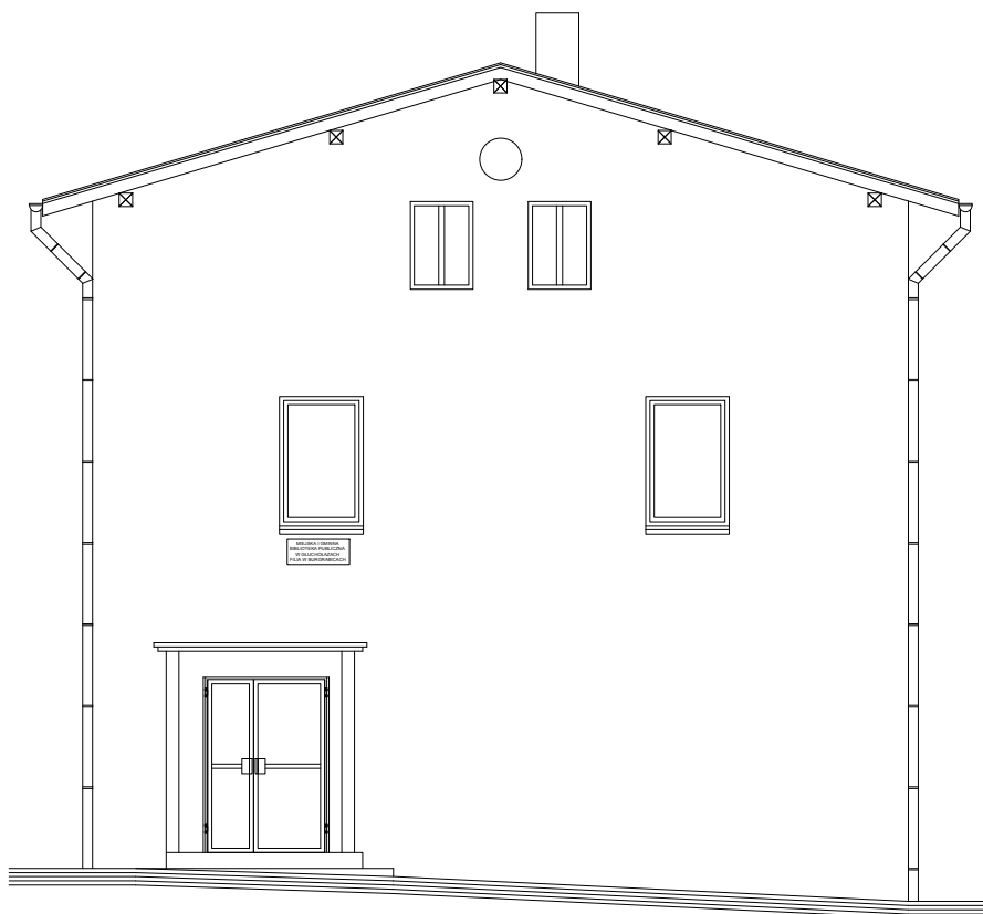
ELEWACJA POŁUDNIOWO-ZACHODNIA
